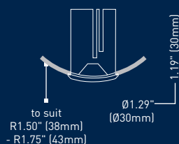
LEDpod XL28 R40
