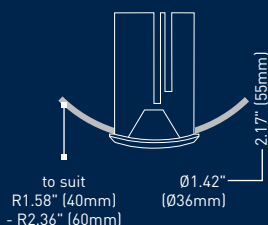
LEDpod XL32 R50
